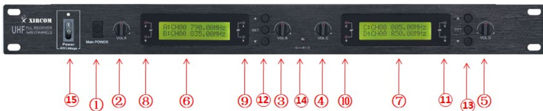
【图 3.2 XC-CG014Z 前面板】
